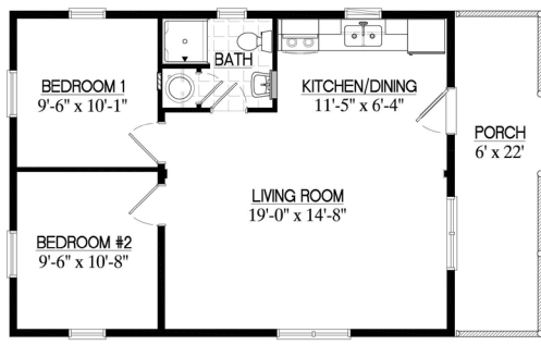
22SR401 22x30 Settler
